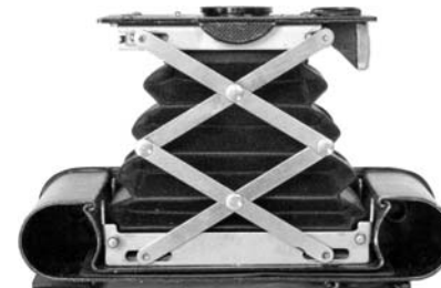
写真10 途中まで伸ばしたVPK。ボディー側、レンズボード側ともにピボットが摺動する。
