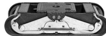
写真2 たたまれた状態。
