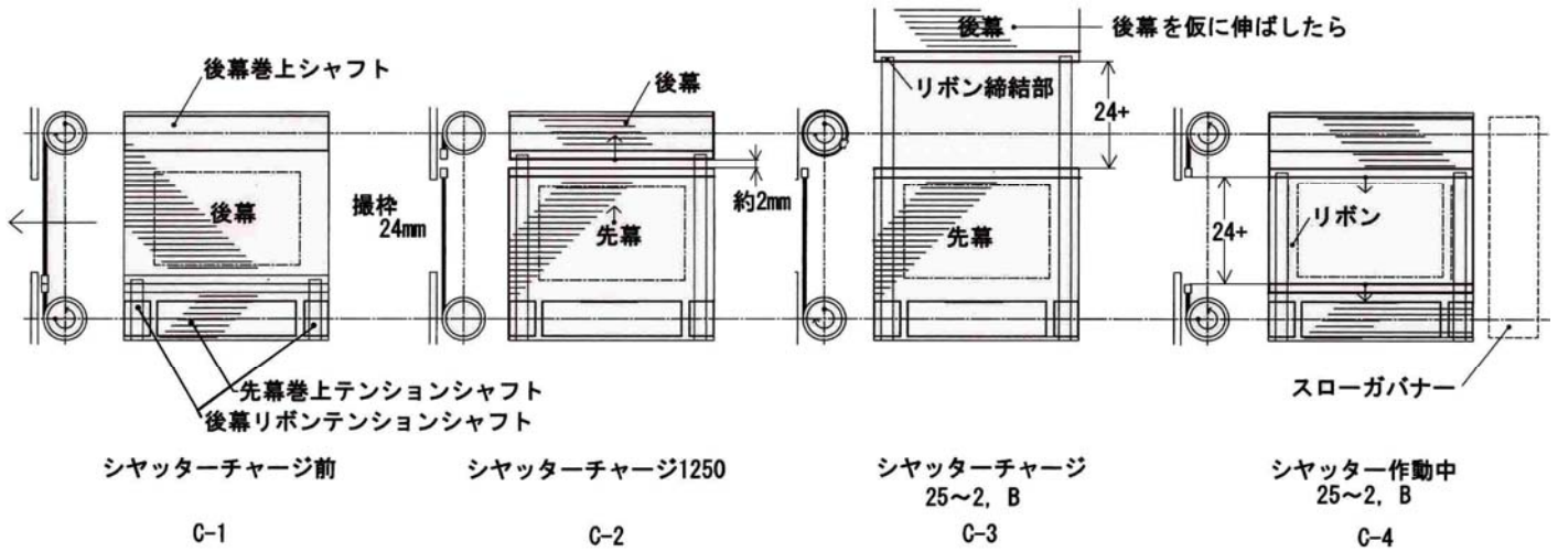
コンタックスのシャッターの作動の様子を示す、左から順に図 C-1シャッターチャージ前、図 C-2高速シャッターチャージ、図 C-3 低速シャッターチャージ 図 C4低速シャッター作動中
