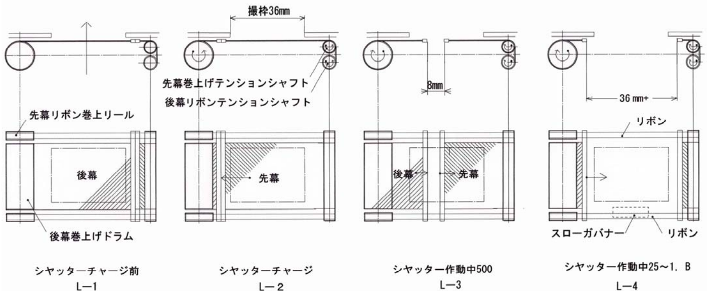
図はライカのシャッターの作動の様子を示す、左から順に図 C-1シャッターチャージ前、図 C-2シャッターチャージ状態、図 C3及びC4 シャッター作動中
