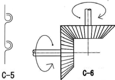
コンタックスの真鍮板の鍍戸式シャッター断面図 (図C-5)と、コンタックスの外部からの回転を直角に曲げるためのベベルギア(図C-6)
