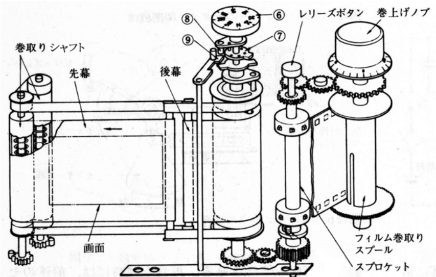
ライカシャッター俯瞰図：後ろ側(フィルム側)から見た図で上の図とは左右が逆転している。(「カメラ技術ハンドブック」：写真工業社、昭和45年7月発行の頁124 図16より一部加工)
